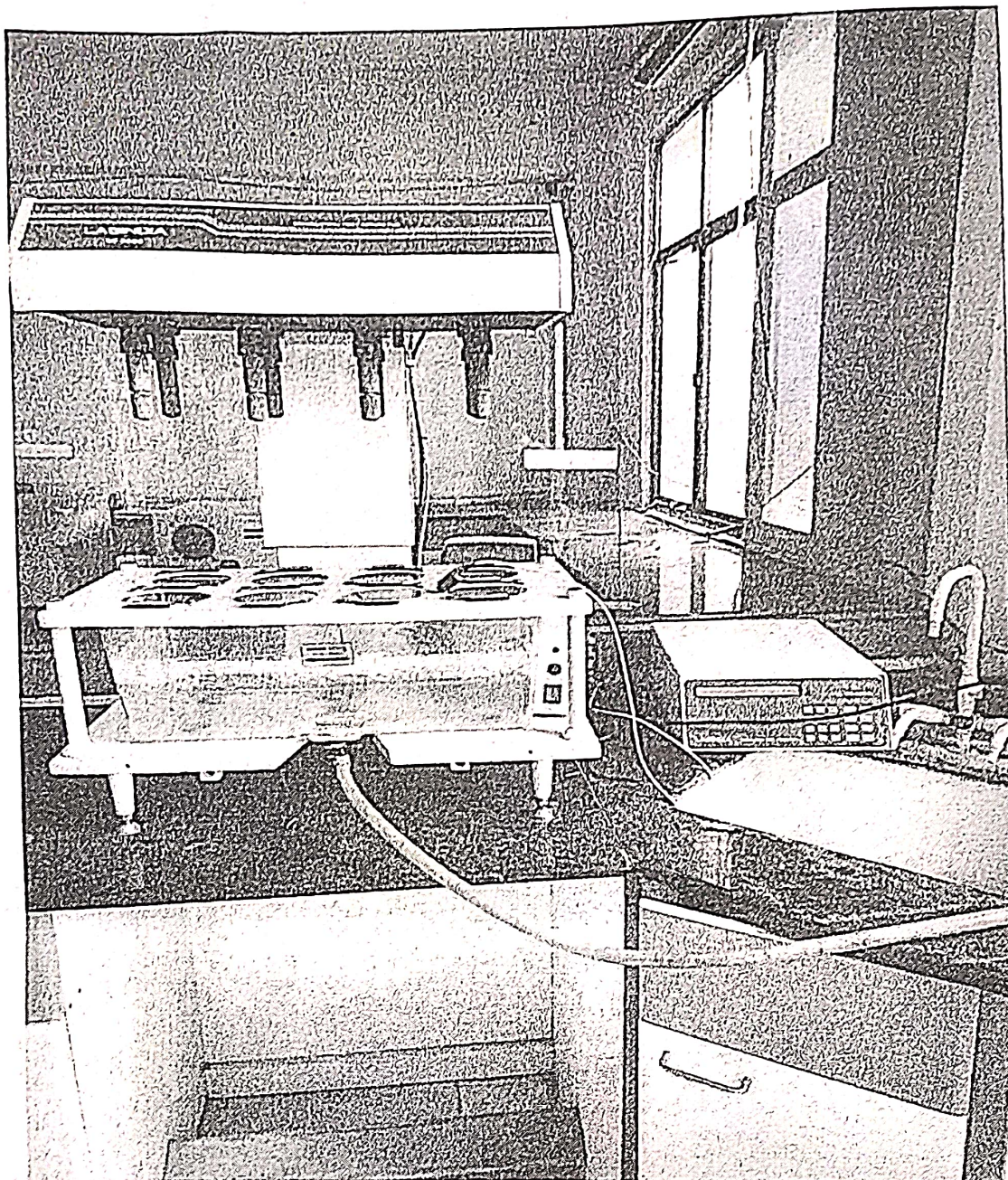
Dissolution Apparatus
